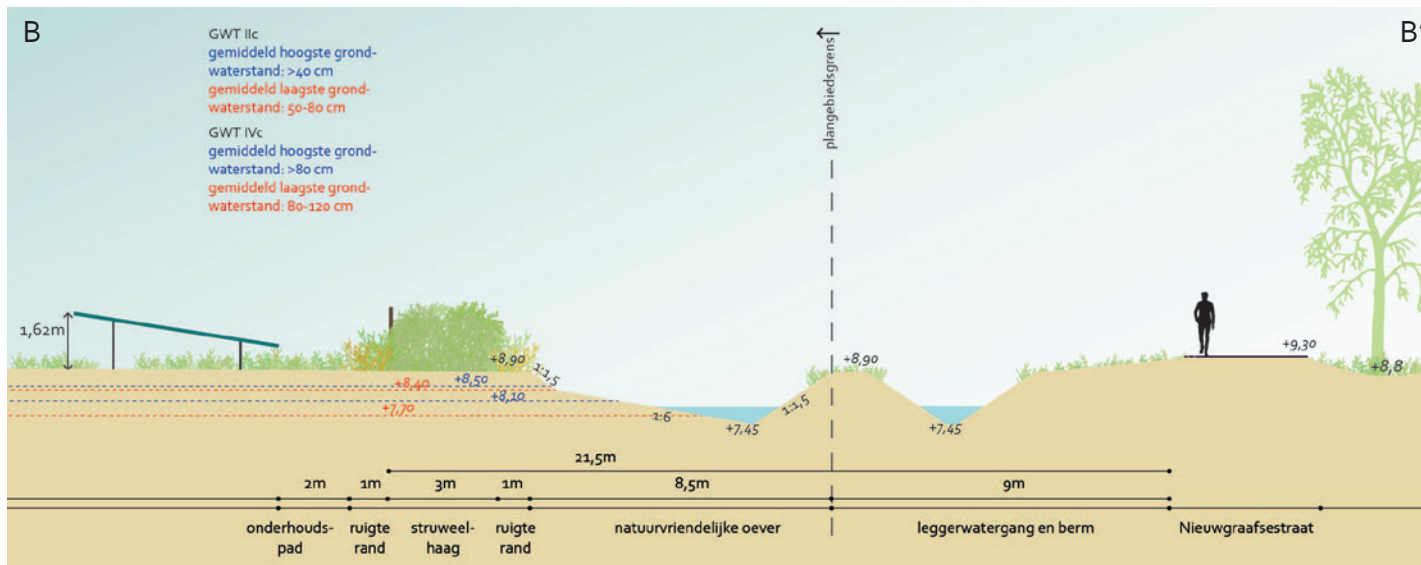
Doorsnede B: toekomstige situatie met natuurvriendelijke oever langs de Nieuwgraafsestraat.
